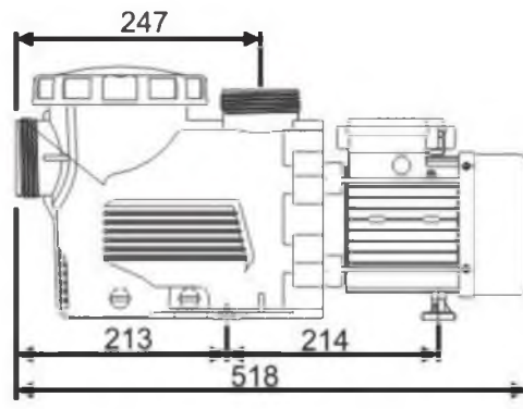
WL-KP1106
