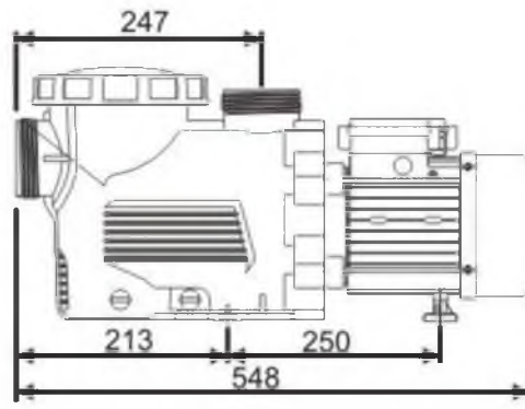
WL-KP1606~WL-KP2206
